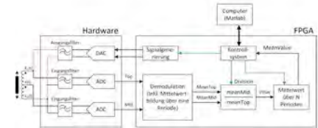
Vereinfachtes Blockdiagramm aus der Designphase des Sensorkonditionierungssystems
