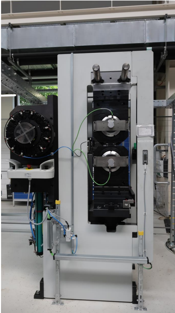
Abb. 1 Kompakt und leistungsfähig: die flexROLLmax kann Bleche bis 0,5 mm Stärke prägen. © Fraunhofer IWU
