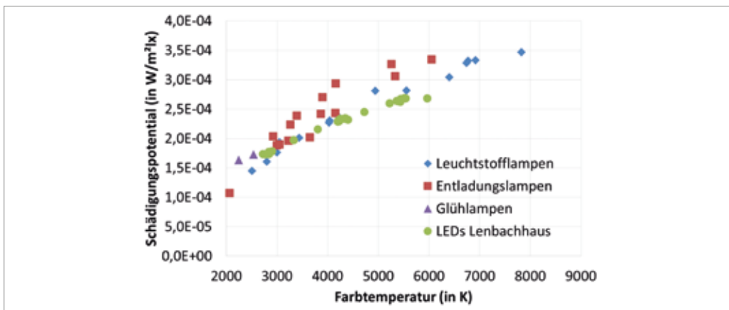
Abbildung 32: Vergleich der Schädigungspotentiale unterschiedlicher Lichtquellen mit den im Lenbachhaus eingesetzten LEDs
