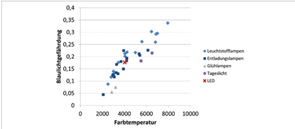
Abbildung 28: Blaulichtgefährdung verschiedener Lichtquellen im Vergleich zu den eingesetzten LEDs © TU Darmstadt
