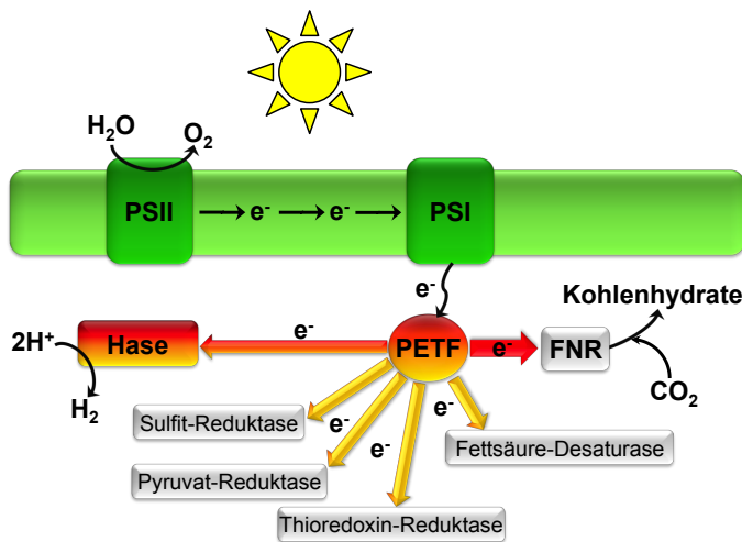
Bild: Elektronentransfer in der Alge C. reinhardtii , der zur Produktion von Wasserstoff oder anderer Stoffe führt. Hase = Hydrogenase. © MPI CEC / RUB
