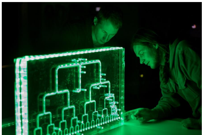
Vermessung einer neuartigen Verteilerstruktur für Kältemittelverdampfer. © Fraunhofer ISE
