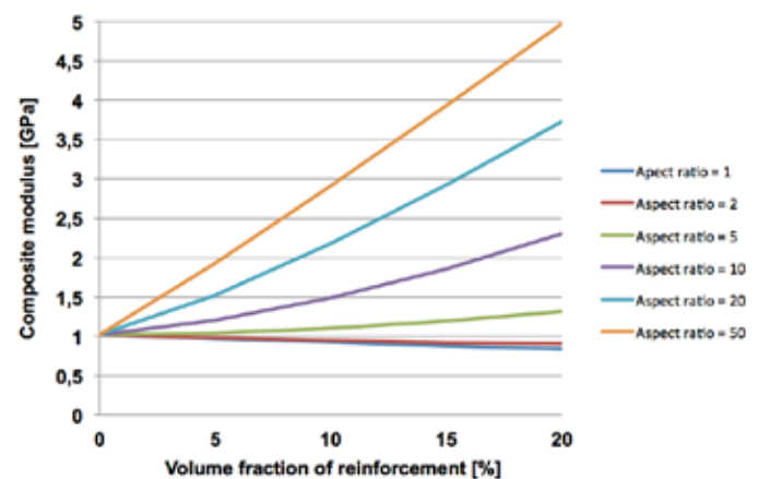
Bild 2a: Einfluss des Längen-Durchmesser-Verhältnisses auf den Elastizitätsmodul
