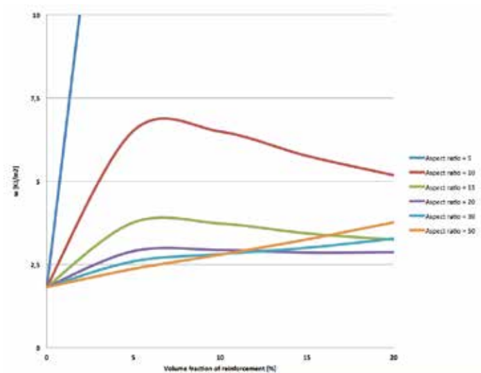
Bild 2b: Einfluss des Längen-Durchmesser-Verhältnisses auf die Schlagarbeit
