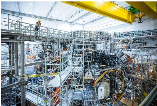
Experimentierhalle mit Wendelstein 7-X in Greifswald (Foto: IPP, Jan Hosan)
