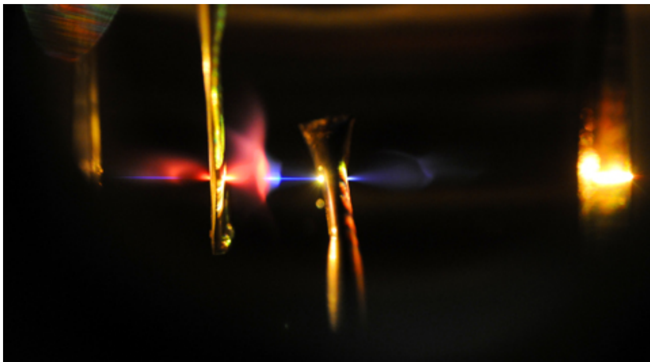
Blick in eine Vakuumkammer, in der Attosekundenpulse erzeugt werden.
