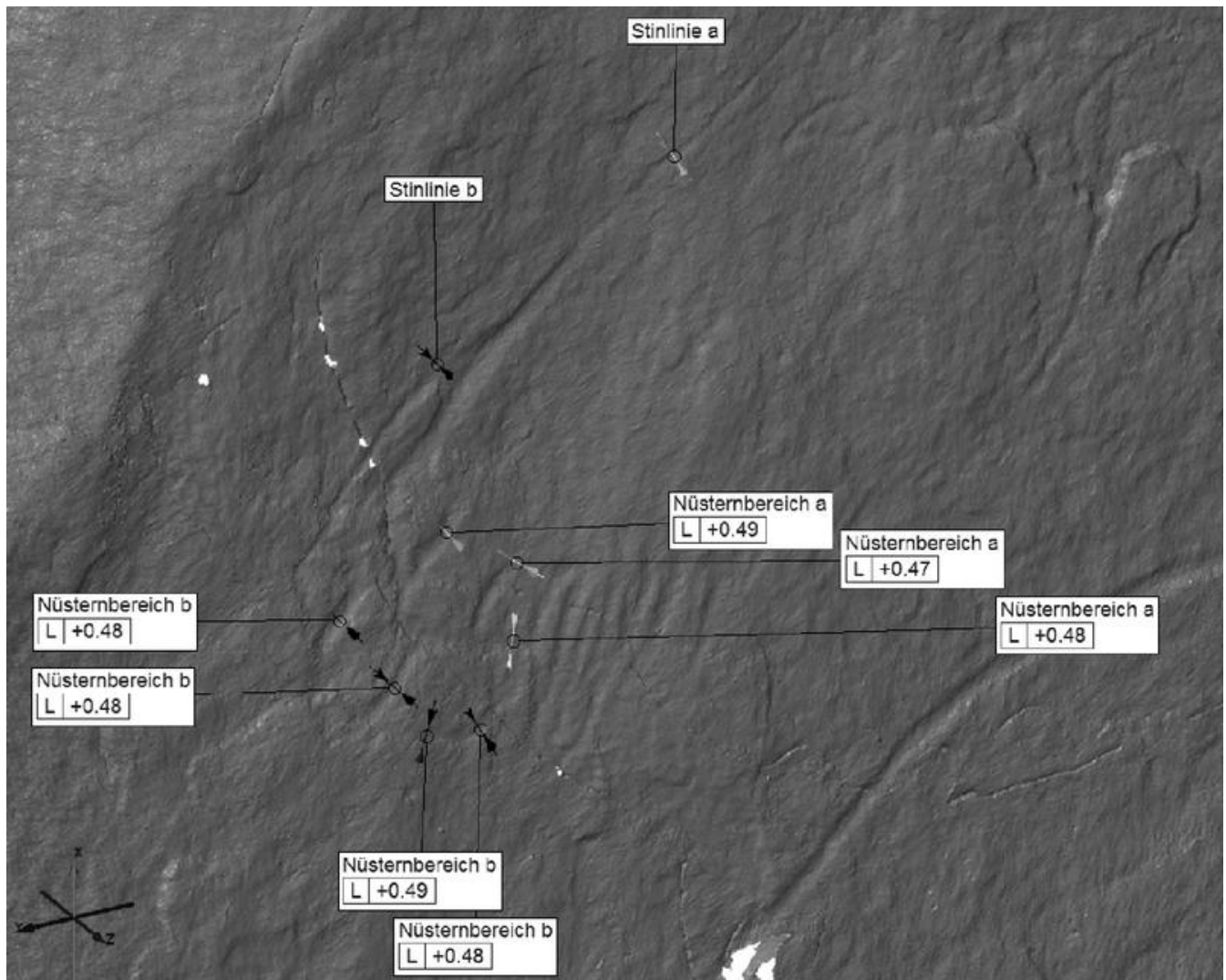
Ausschnitt eines Detailscans der Pferdeköpfs von Platte 59. Angegeben sind die Linienbreiten der Gravierungen an ausgewählten Messpunkten des 3D-Scans
