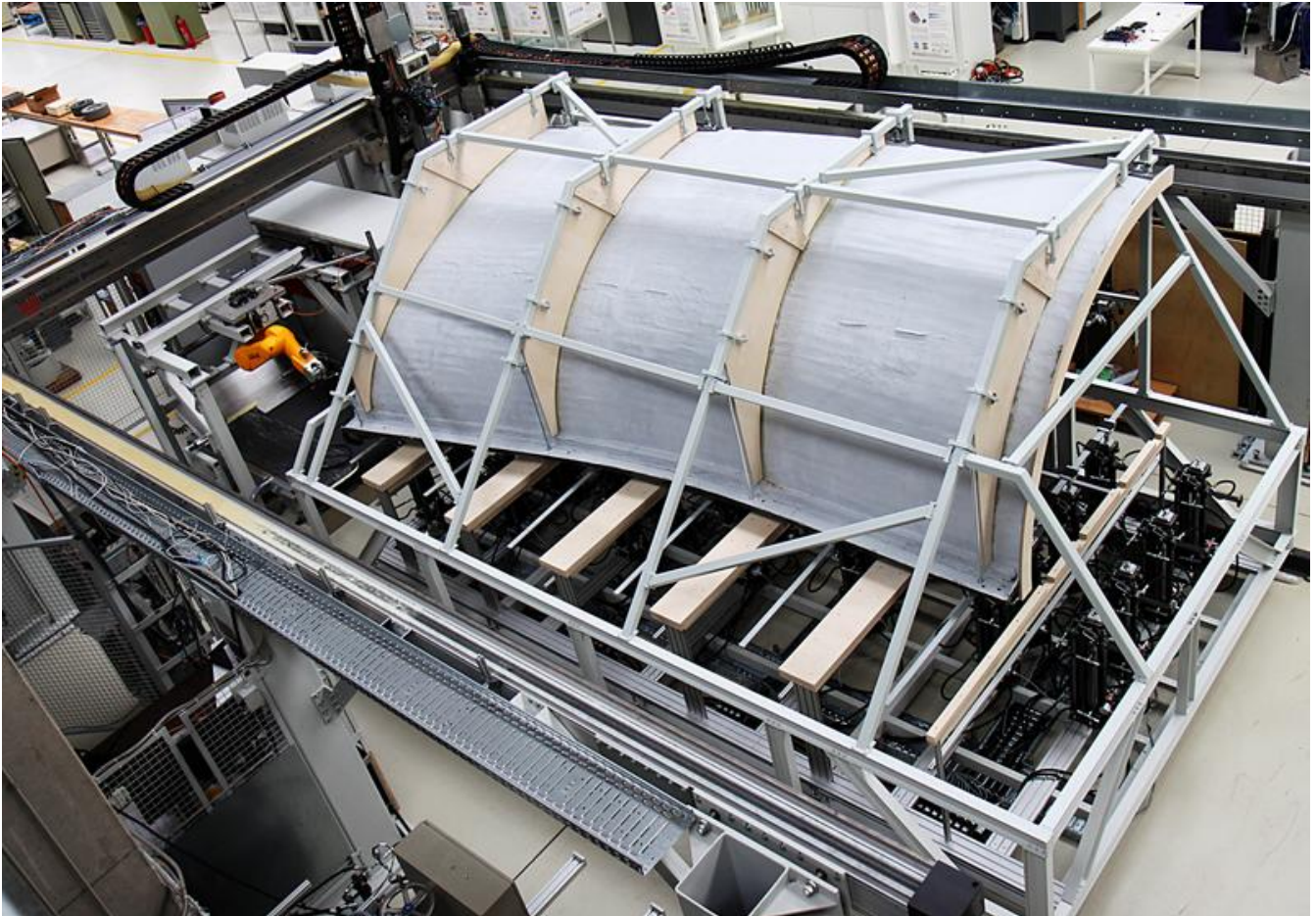
Sicht auf Gesamtforschungsanlage des Instituts für integrierte Produktentwicklung aus dem Projekt mapretec. "Foto: Jan-Hendrik Ohlendorf / BIK"
