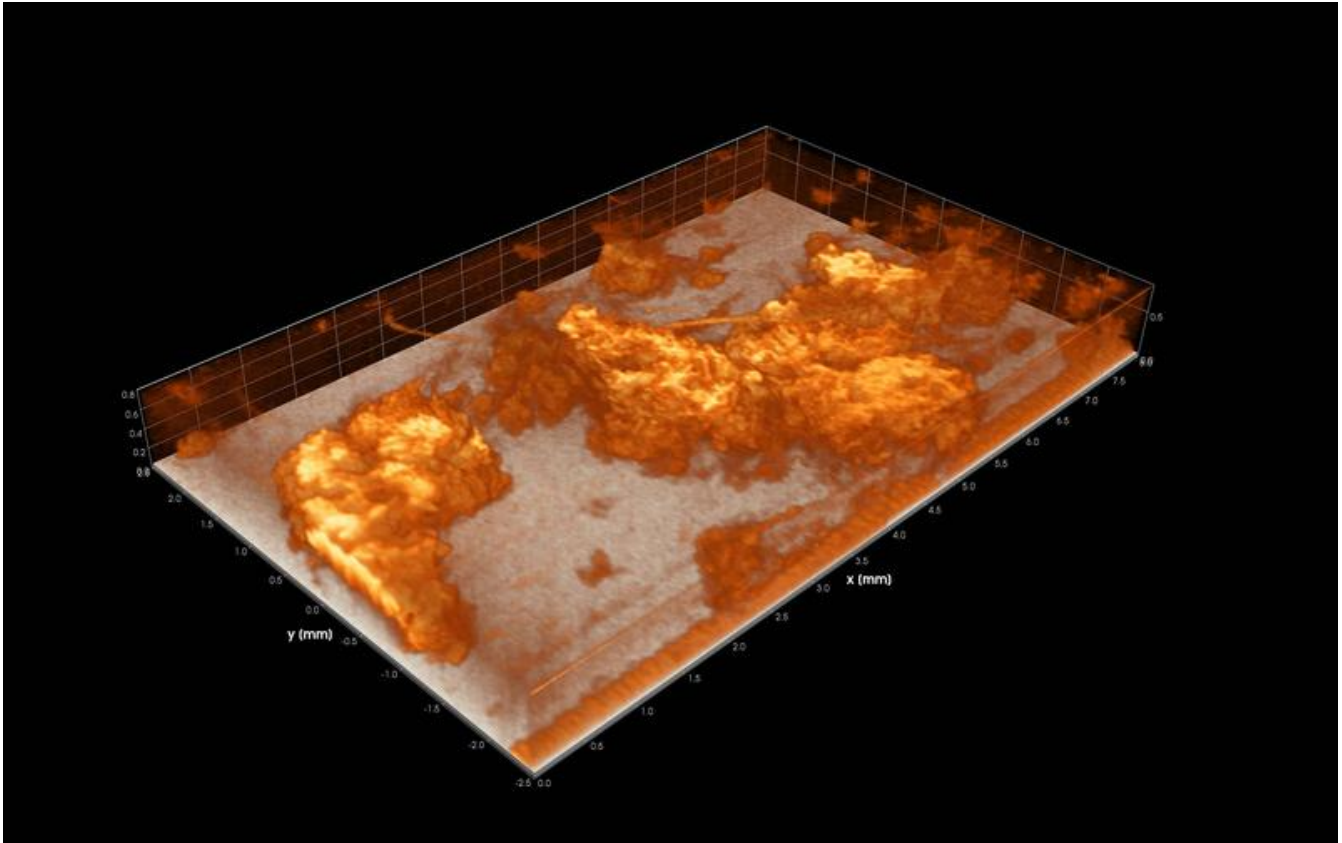
Biofilm auf der Anode (Boden) der Brennstoffzelle: Mit optischer Kohärenztomographie machen Forscher des KIT die mikrobiellen Biofilme sichtbar, die elektrische Energie erzeugen Grafik: Michael Wagner, KIT
