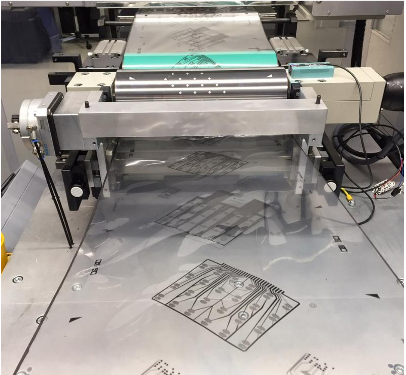
Endlosfolie mit gedruckten Biosensoren: Fraunhofer hat ein günstiges Rolle-zu-Rolle-Verfahren entwickelt. Fraunhofer IBMT
