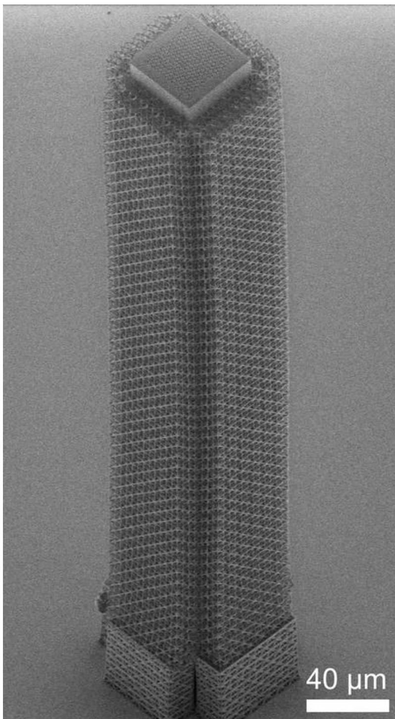
Zu sehen ist ein photonischer Quantensimulator. Die eigentliche Struktur befindet sich im inneren Block und ist selbst unter dieser Vergrößerung nicht sichtbar. Foto: Arbeitsgruppe von Freymann
