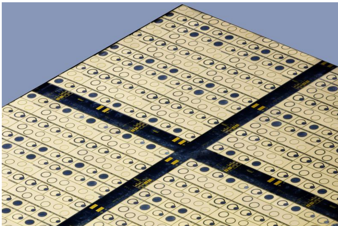
Galliumoxid-Chip mit Transistor- und Messstrukturen, hergestellt am FBH mittels Projektionsbelichtung FBH/schurian.com
