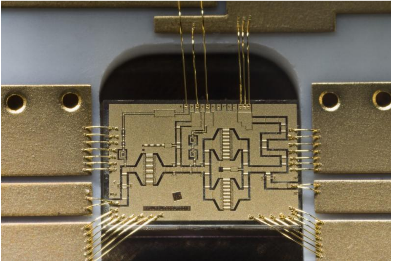
Galliumnitrid-Verstärker aus einem früheren Projekt des FBH. Im Projekt ForMikro-LeitBAN soll die Technologie für Millimeterwellen auf Aluminiumnitrid übertragen werden. FBH/schurian.com
