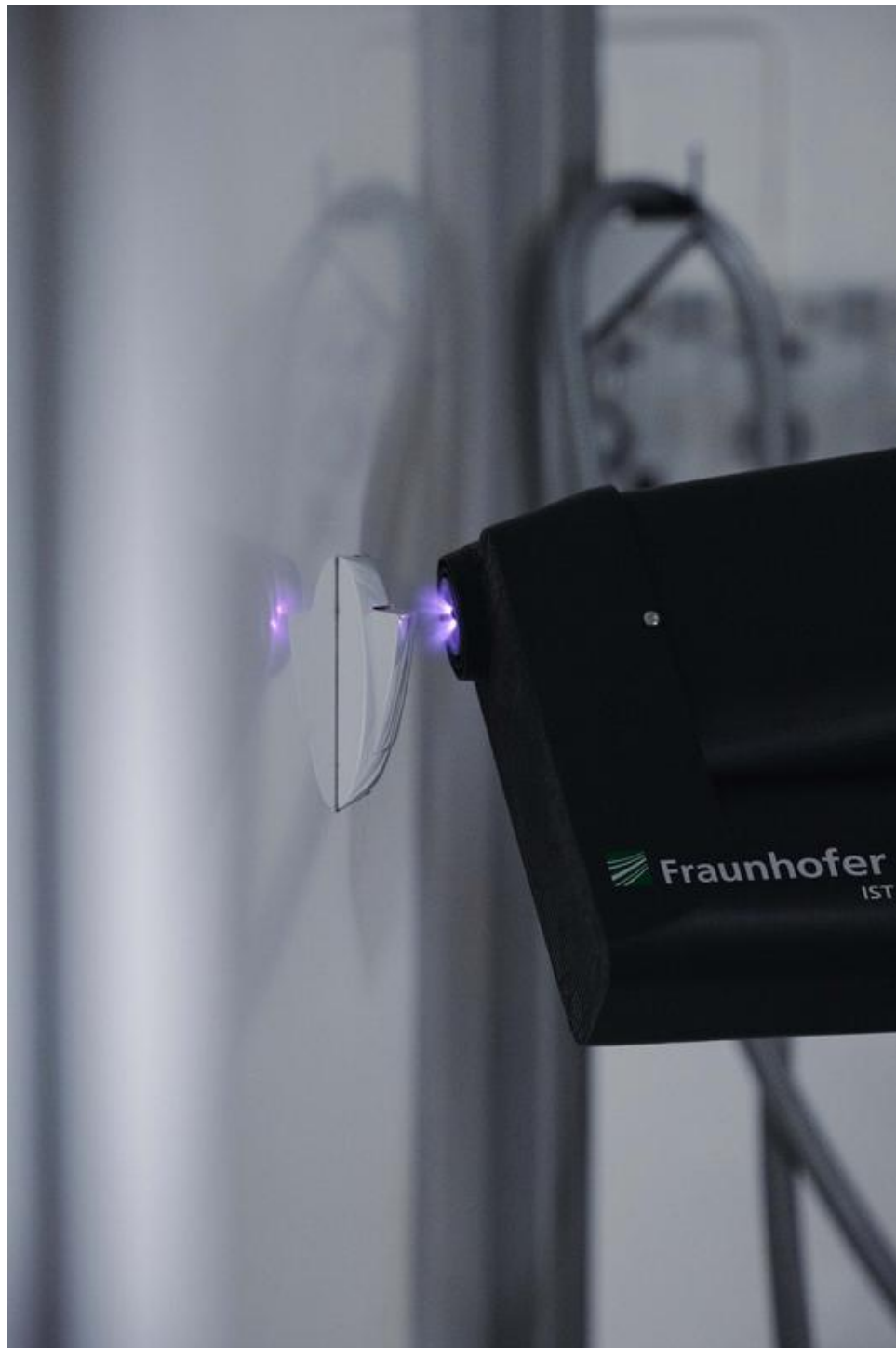
Modulare Plasmaquelle zur Reinigung und Desinfektion von Oberflächen. © Fraunhofer IST, Paul Kurze
