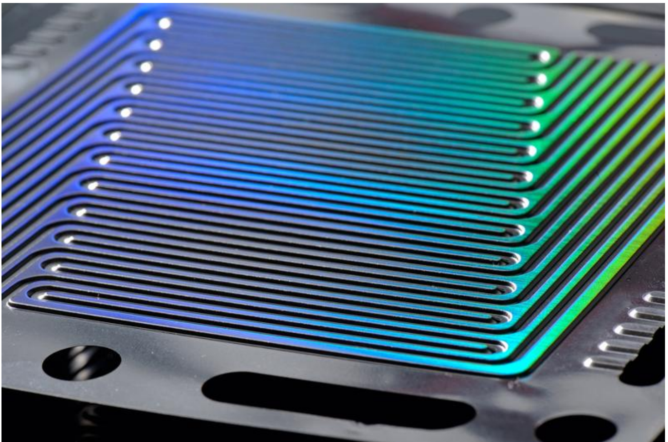
Mittels UKP-Lasermikrostrukturierung funktionalisierte Bipolarplatte (Design der Bipolarplatte: Dana Victor Reinz). Fraunhofer ILT, Aachen.
