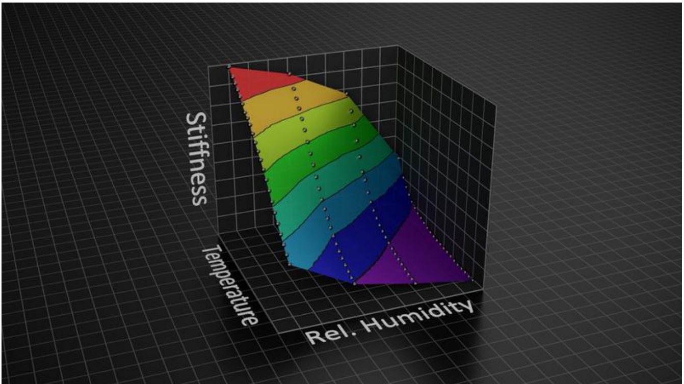
Abhängigkeit der Steifigkeit von äußeren Umweltbedingungen, wie Temperatur und relativer Luftfeuchte F. Sterl Universität Stuttgart, FSM-Labor
