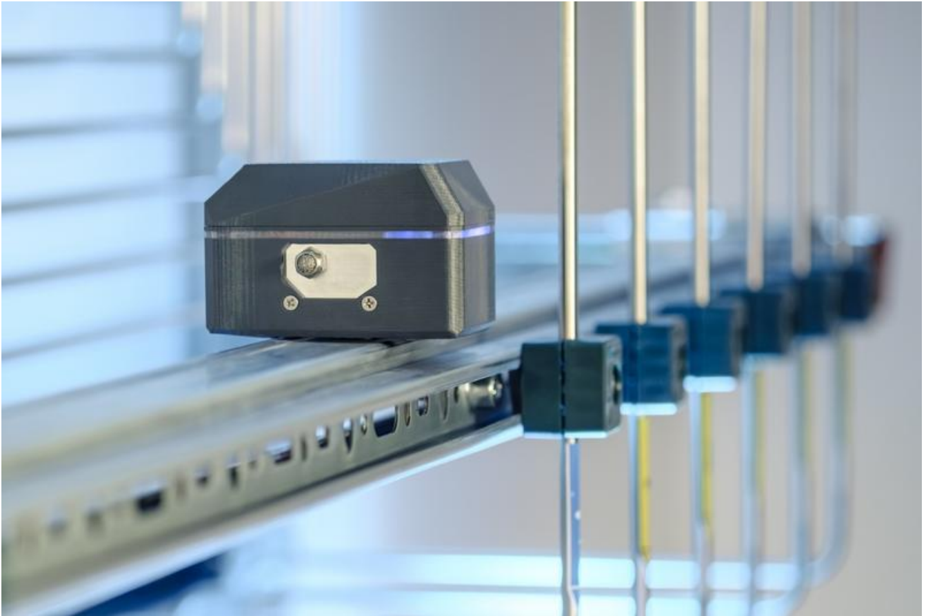
Mit dem Ultraschallsensor können Wasserstoff-Behälter, -Leitungen oder -Verbindungsstücke überwacht werden. © Fraunhofer IPM
