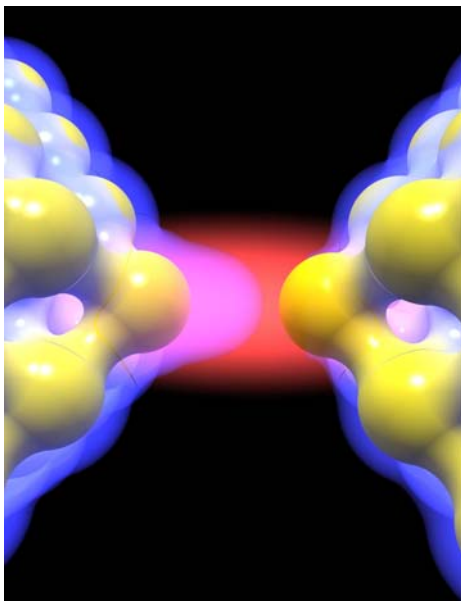
Tausendfach verstärktes elektromagnetisches Feld in der Lücke zwischen zwei Goldnanostrukturen. Die schematische Darstellung zeigt Goldatome und ihre chemischen Bindungen (gelb), die Elektronendichte (blau) und das erhöhte elektromagnetische Feld (rot). (Abbildung: Daniel R. Ward)
