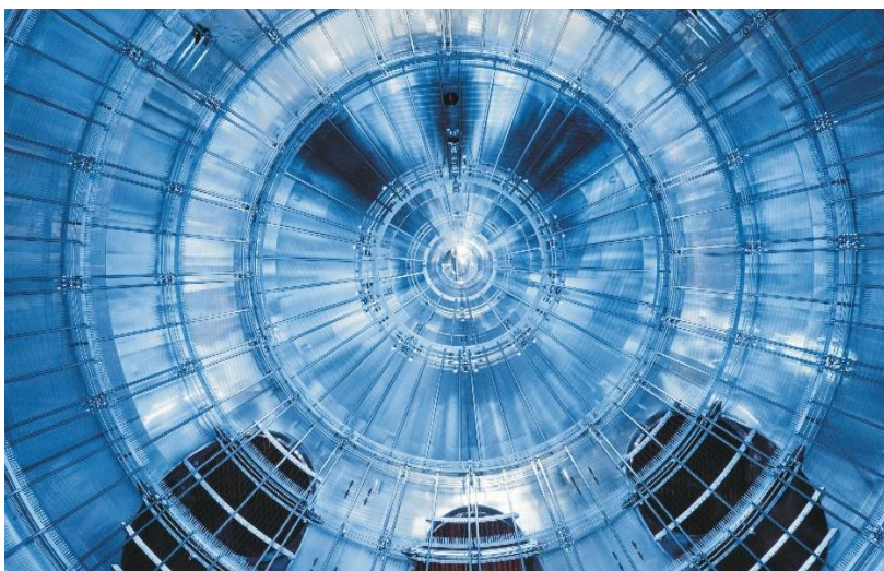
Dem leichtesten Teilchen des Universums ist das KIT mit der riesigen Neutrinowaage KATRIN am Campus Nord auf der Spur. (Bild: M. Breig/KIT)
