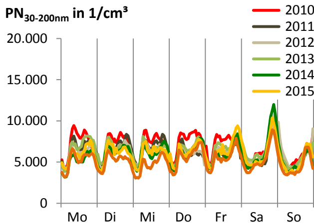
Abbildung 24: Mittlerer Tagesgang der Woche an der verkehrsnahen Messstation Leipzig-Eisenbahnstraße (LEI) für PN_{30-200nm} und Ruß- BC_{PM1} von 2010 bis 2016
