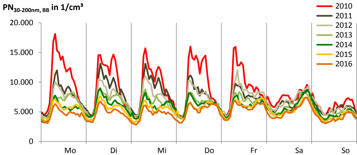
Abbildung 11: Mittlerer Tagesgang der Woche für die Konzentrationen von Ruß und Partikel von 30 bis 200 nm an Leipzig-Mitte vor Einführung der Umweltzone 2010 und in den Jahren danach bis 2016
