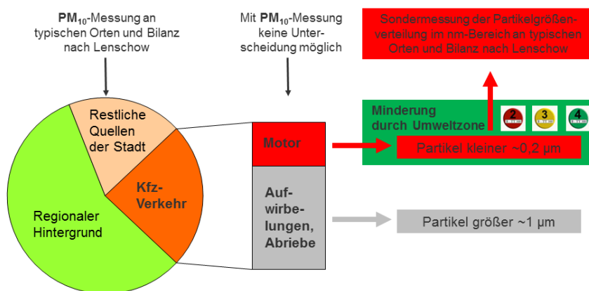
Abbildung 4: Schema der Verursacheranalyse für eine verkehrsnahen PM_{10} -Belastung mit Ermittlung des Immissionsanteils Motor durch die Immissionsmessung der Partikelgrößenverteilung
