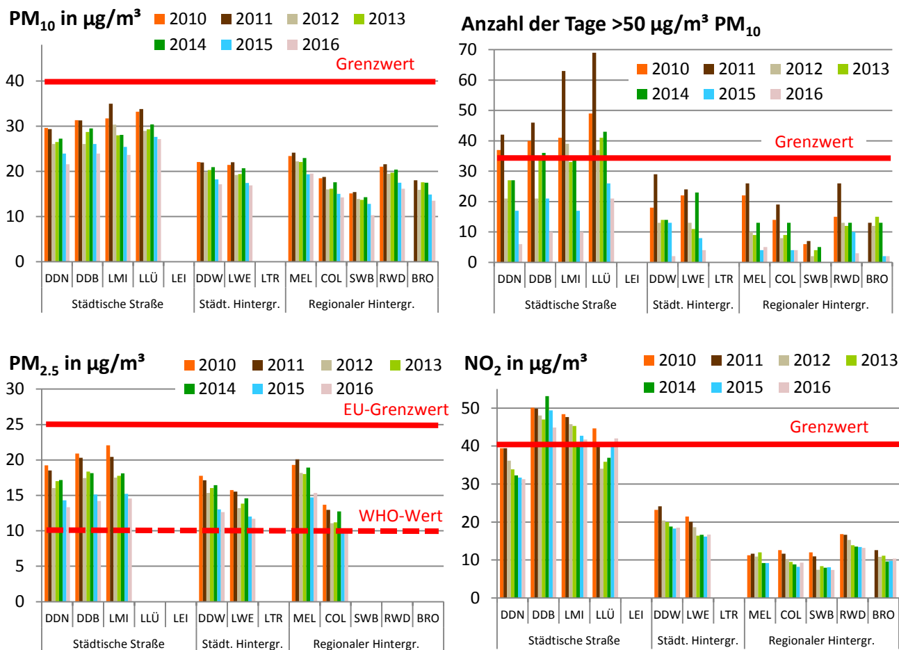
Abbildung 17: Ergebnisse der Messung für PM 10 , PM 2.5 und NO 2 für die Jahresmittelwerte von 2010 bis 2016 und dessen Relation zum jeweiligen Grenzwert zum Schutz der menschlichen Gesundheit
