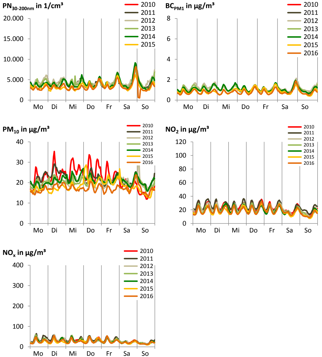
Abbildung 25: Mittlerer Tagesgang der Woche an der städtischen Hintergrund-Messstation Dresden-Winkelmannstraße (DDW) für PN 30-200nm , Ruß-BC PM1 , PM 10 , NO 2 und NO x von 2010 bis 2016
