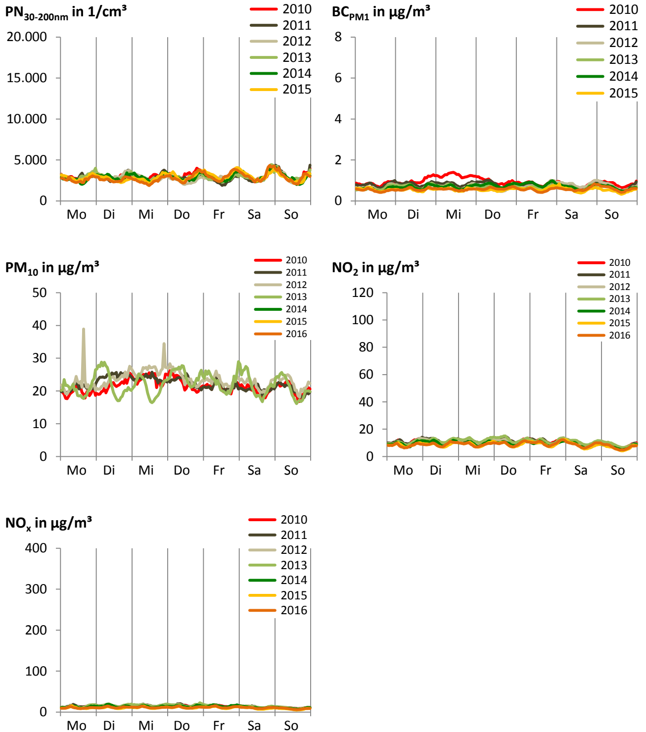
Abbildung 28: Mittlerer Tagesgang der Woche an der regionalen Hintergrund-Messstation Melpitz (MEL) für PN 30-200nm , Ruß-BC PM1 , PM 10 , NO 2 und NO x von 2010 bis 2016
