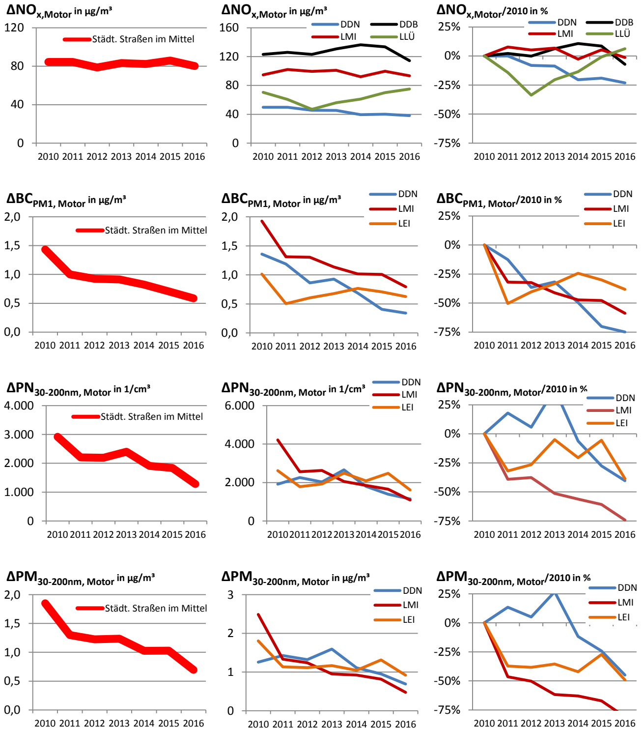
Abbildung 13: Entwicklung des Immissionsanteils Motor am Stationstyp „Städtische Straße“ und an den einzelnen straßennahen Stationen für das Gas \text{NO}_x und die Partikel \text{BC}_{\text{PM1}} , \text{PN}_{30-200\text{nm}} und \text{PM}_{30-200\text{nm}} von 2010 bis 2016
