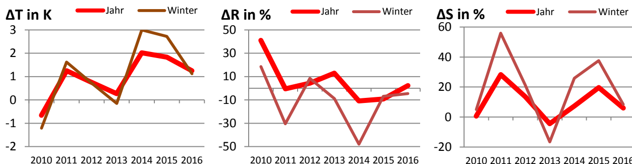
Abbildung 8: Abweichungen meteorologischer Parameter \Delta T , \Delta R und \Delta S von 2010 bis 2016 gegenüber dem Referenzzeitraum 1961 bis 1990
