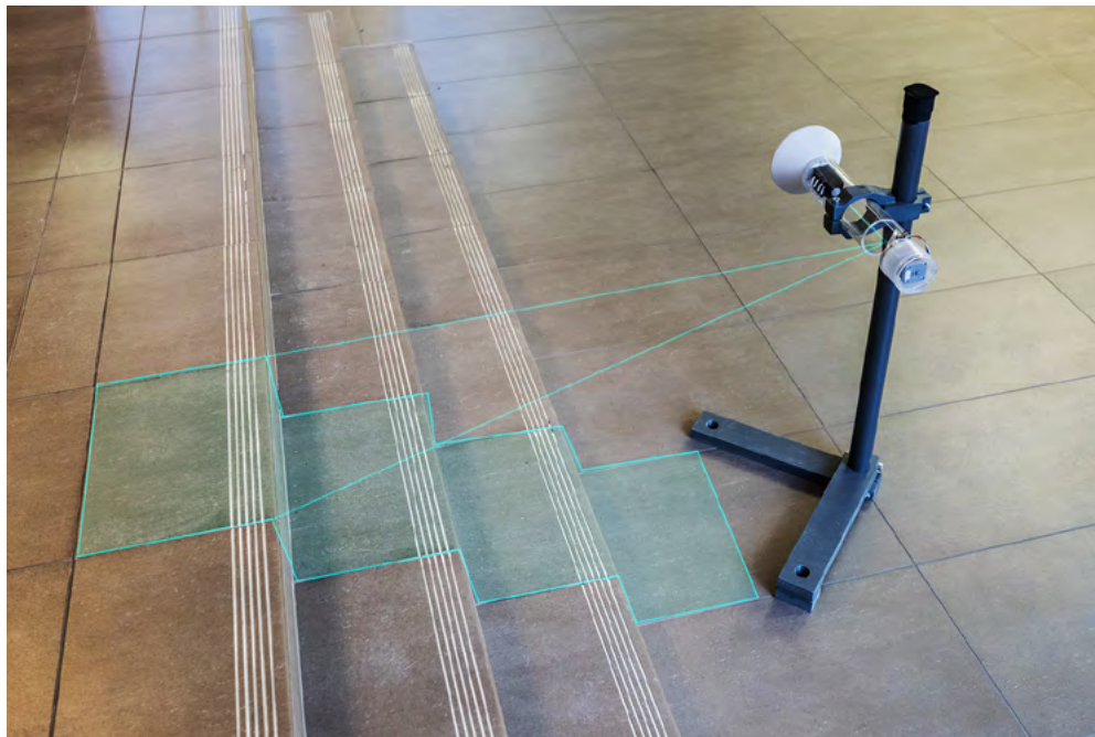
Integrierter 2D-Radarscanner des Fraunhofer IPA zur Umfeld-Erkennung. (Quelle: Fraunhofer IPA, Foto: Rainer Bez)
