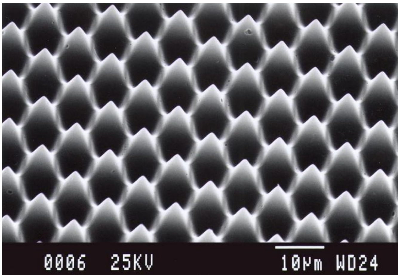
Oberfläche mit selbstreinigender Wirkung unter dem Rasterelektronenmikroskop
