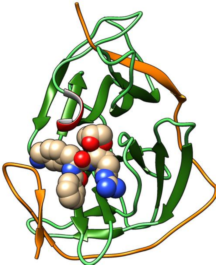
Dreidimensionale Struktur der Zikavirus-Protease
