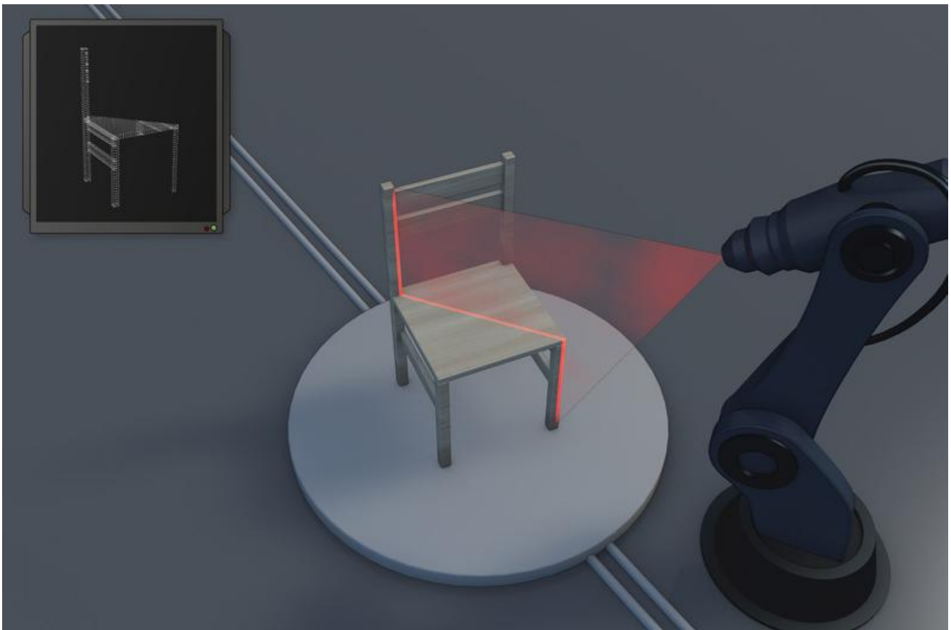
Graphische schematische Darstellung des 3D-Scans am Beispiel eines Stuhls. © Fraunhofer ITWM
