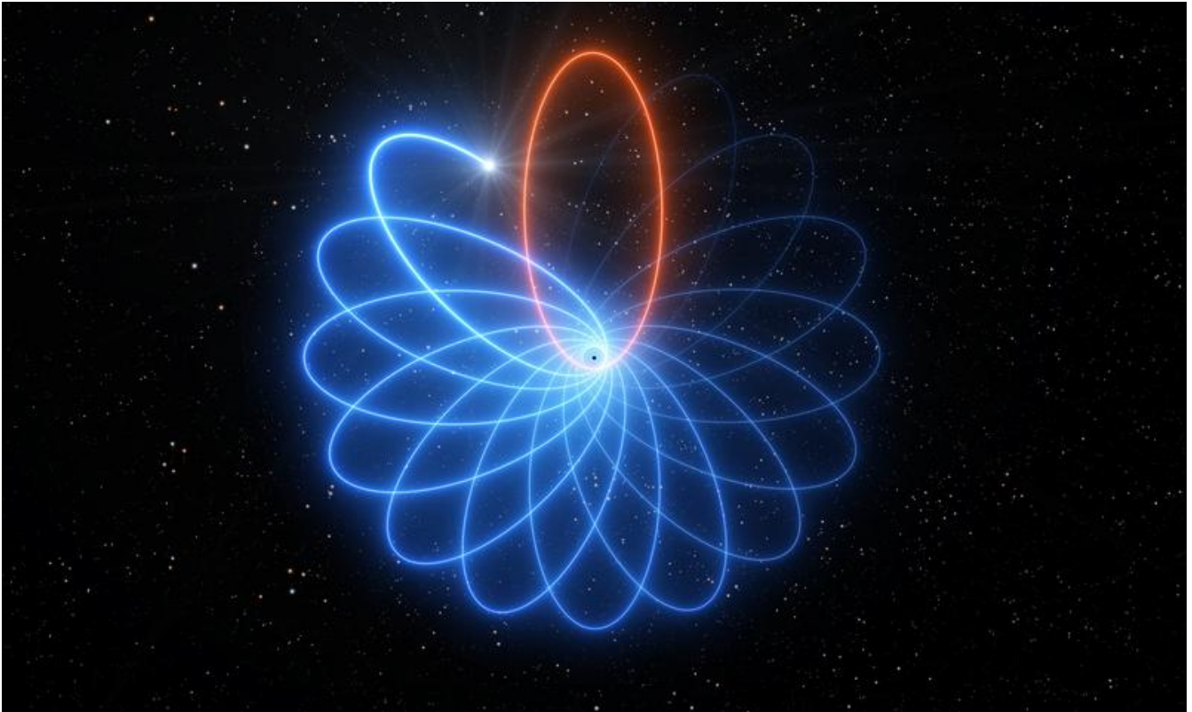
Künstlerische Darstellung der Schwarzschild-Präzession einer Stern-Umlaufbahn um das zentrale Schwarze Loch unserer Milchstraße - der relativistische Effekt ist übertrieben dargestellt Bild: ESO/L. Calçada
