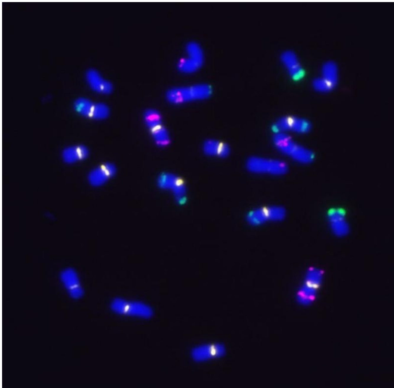
Mais Metaphase-Chromosomen nach Fluoreszenz-in-situ-Hybridisierung (FISH)
