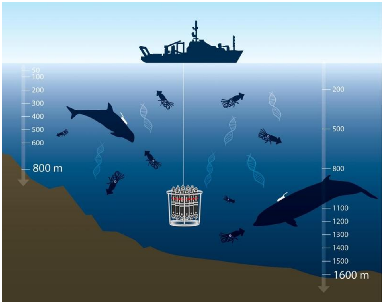
Schematisches Diagramm zur Illustration der Probenahme von Tintenfisch-Umgebungs-DNA (eDNA) in den Nahrungsgebieten von Risso-Delfinen (links) und Cuvier-Schnabelwalen (rechts).
