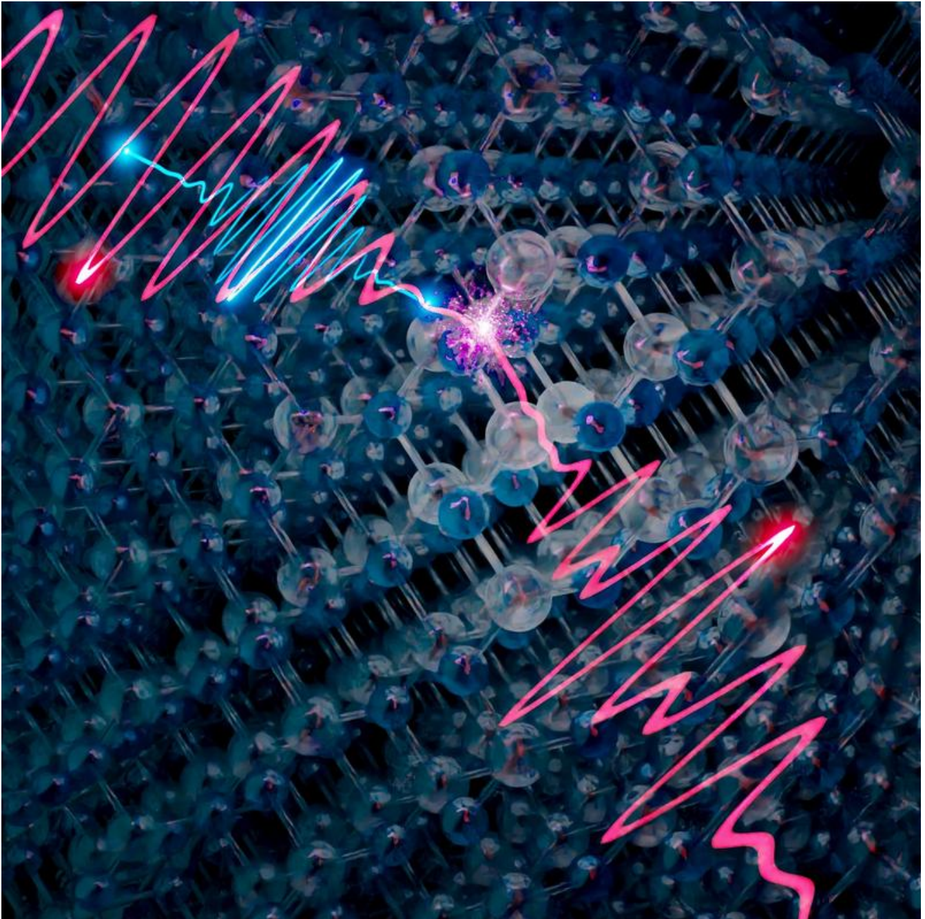
Ein nah-infraroter Laserpuls (blau) regt einen Halbleiter an. Die sich entfaltende ultraschnelle Dynamik wird mittels feldaufgelöster Spektroskopie untersucht. Änderungen in der Wellenform eines reflektierten mittelinfraroten Lichtfeldes (rot) RMT Bergues
