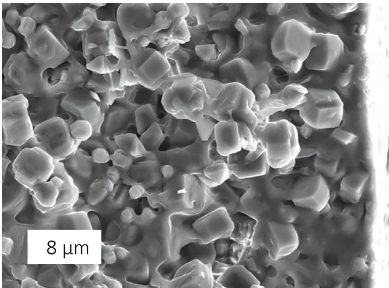
Rasterelektronenmikroskop-Aufnahme einer Kompositmembran. © Fraunhofer IKTS
