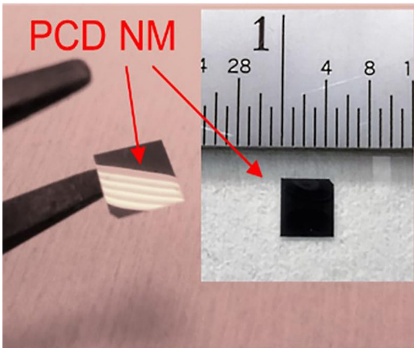
Fotos von freistehenden polykristallinen Diamant-Nanomembranen © Fraunhofer USA, Center Midwest
